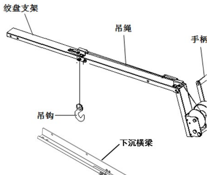
图2-18 风机升降组件（绞盘方式）
