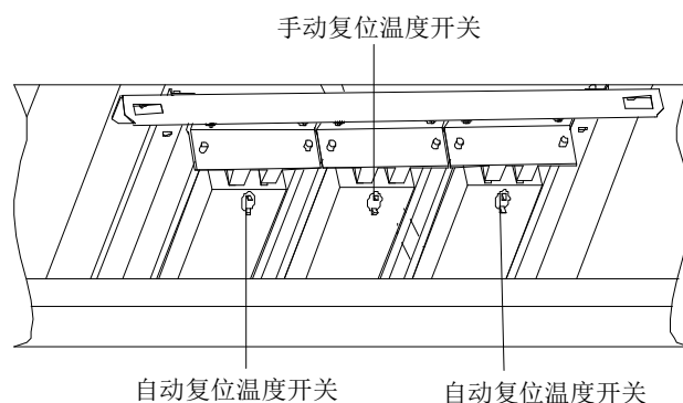
图5-2 PTC 电加热
